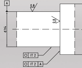
gehäuse und schaft housing and shaft
