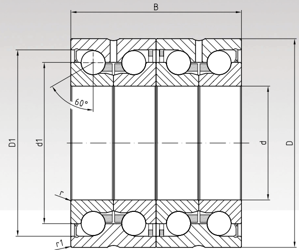
gepaarte version 2ap / paired version 2ap
